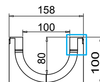
VISTA FRONTALE
