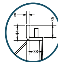
PART. TELAIO
