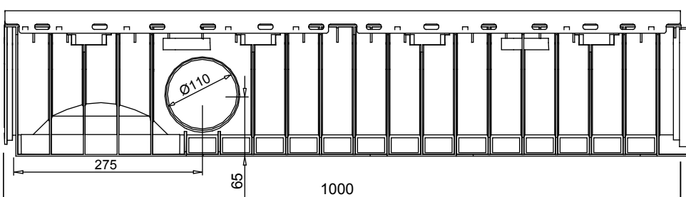
VISTA LATERALE
