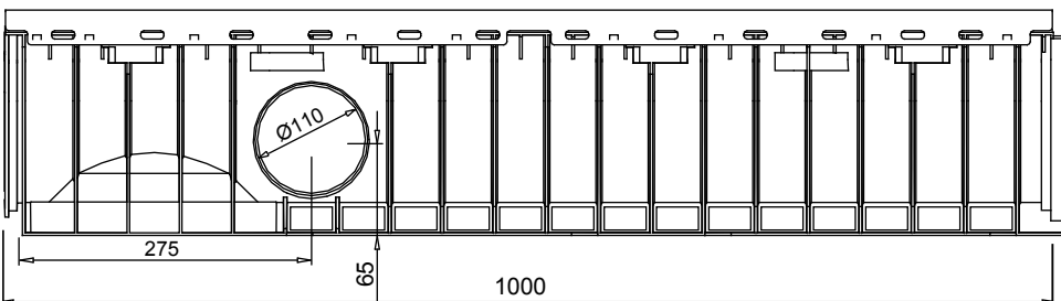
VISTA LATERALE
