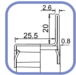
PART. SEZIONE
