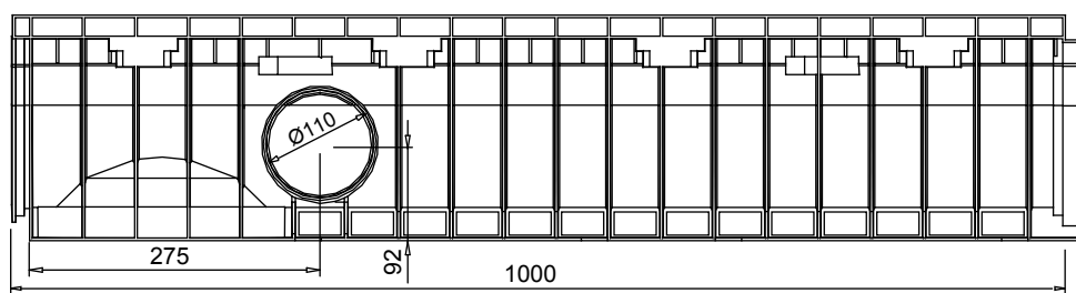
VISTA LATERALE
