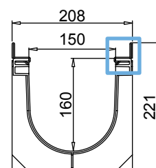
SEZIONE
