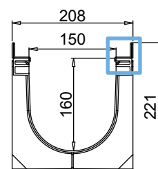
SEZIONE
