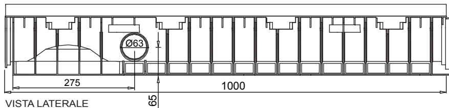
VISTA LATERALE
