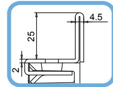
PART. SEZIONE
