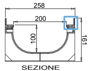
SEZIONE
