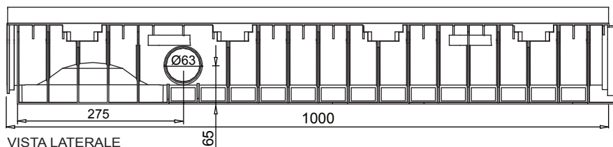
VISTA LATERALE
