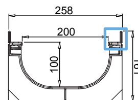
SEZIONE
