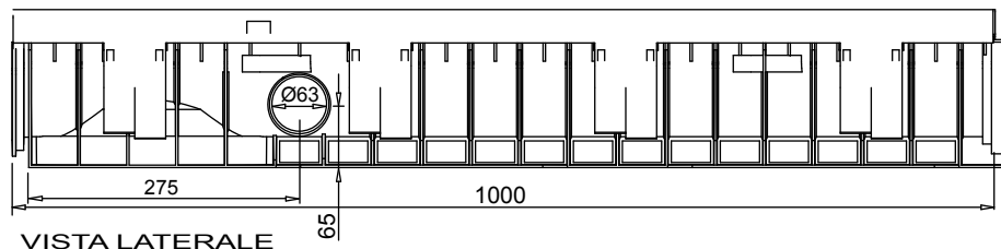
VISTA LATERALE
