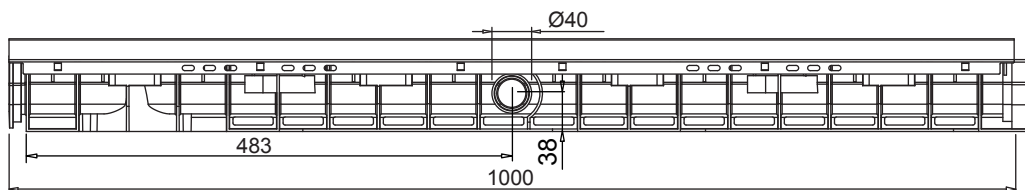
VISTA LATERALE
