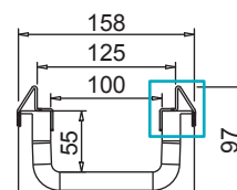
VISTA FRONTALE
